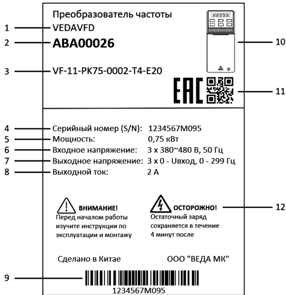
Рисунок 1.3-1 – Пример маркировки преобразователя частоты
