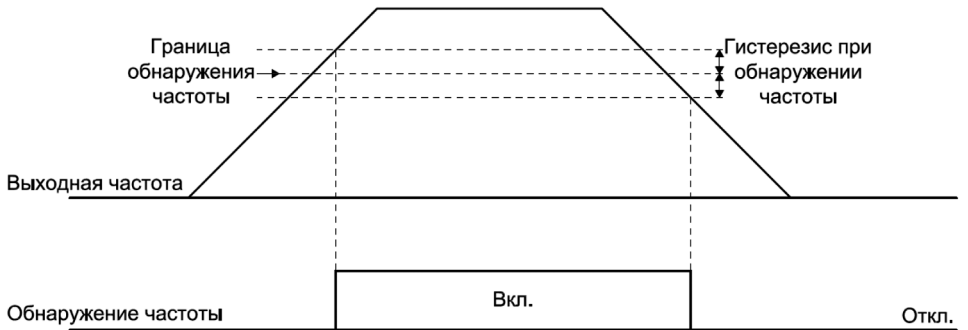
Рисунок 10.10-1 – Граница и гистерезис обнаружения выходной частоты (функций 9 и 10 параметров F06.21-F06.22)
