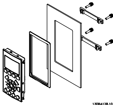
Рисунок 3.24: Монтажный комплект для LCP, включающий графическую панель LCP, крепеж, кабель (3 м) и прокладку
