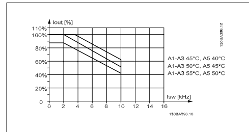
Рисунок 3.4: Снижение тока I_{out} для различных значений T_{amb, max} для корпуса А, при использовании модели коммутации SFAVM и длине кабеля до 10 м.
