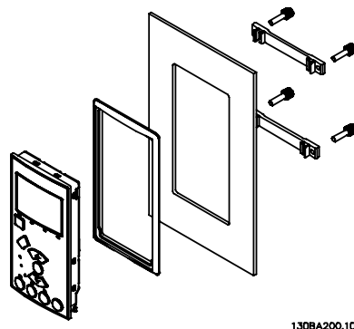
Рисунок 3.25: Монтажный комплект для LCP, содержащий цифровую панель LCP, крепеж и прокладку
