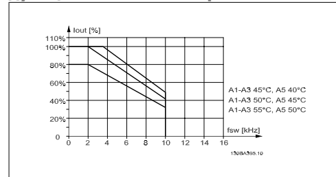
Рисунок 3.2: Снижение тока I_{out} для различных значений T_{amb, max} для корпуса А при использовании модели коммутации 60 SFAVM
