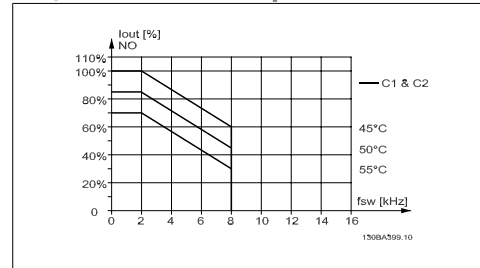
Рисунок 3.8: Снижение тока I_{out} для различных значений T_{AMB, MAX} для корпуса С при использовании модели коммутации SFAVM в режиме нормального крутящего момента (перегрузка по крутящему моменту 110 %).
