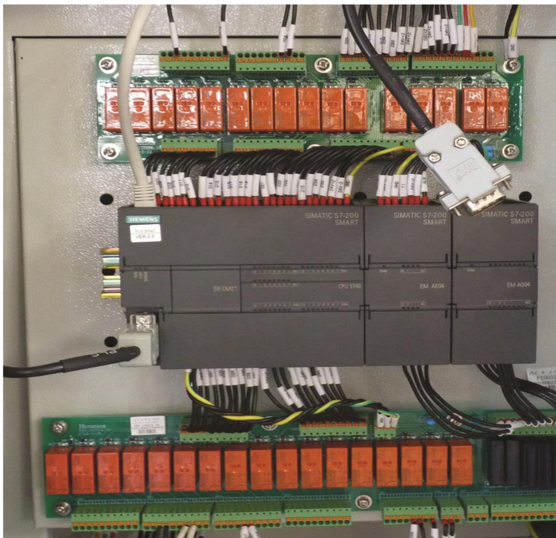
Рис. 3.2 - Секция управления
