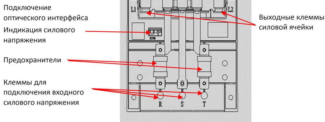
Рис. 1.9 - Внешний вид силовой ячейки с передней стороны
