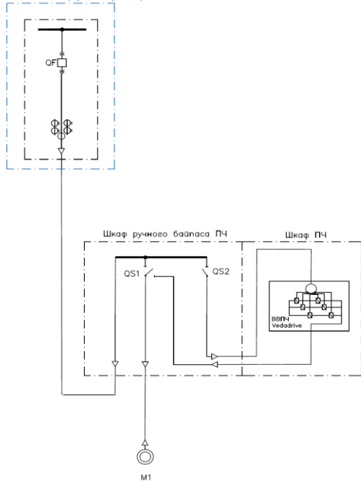
Рис. 6.3 - Схема ручного байпаса
