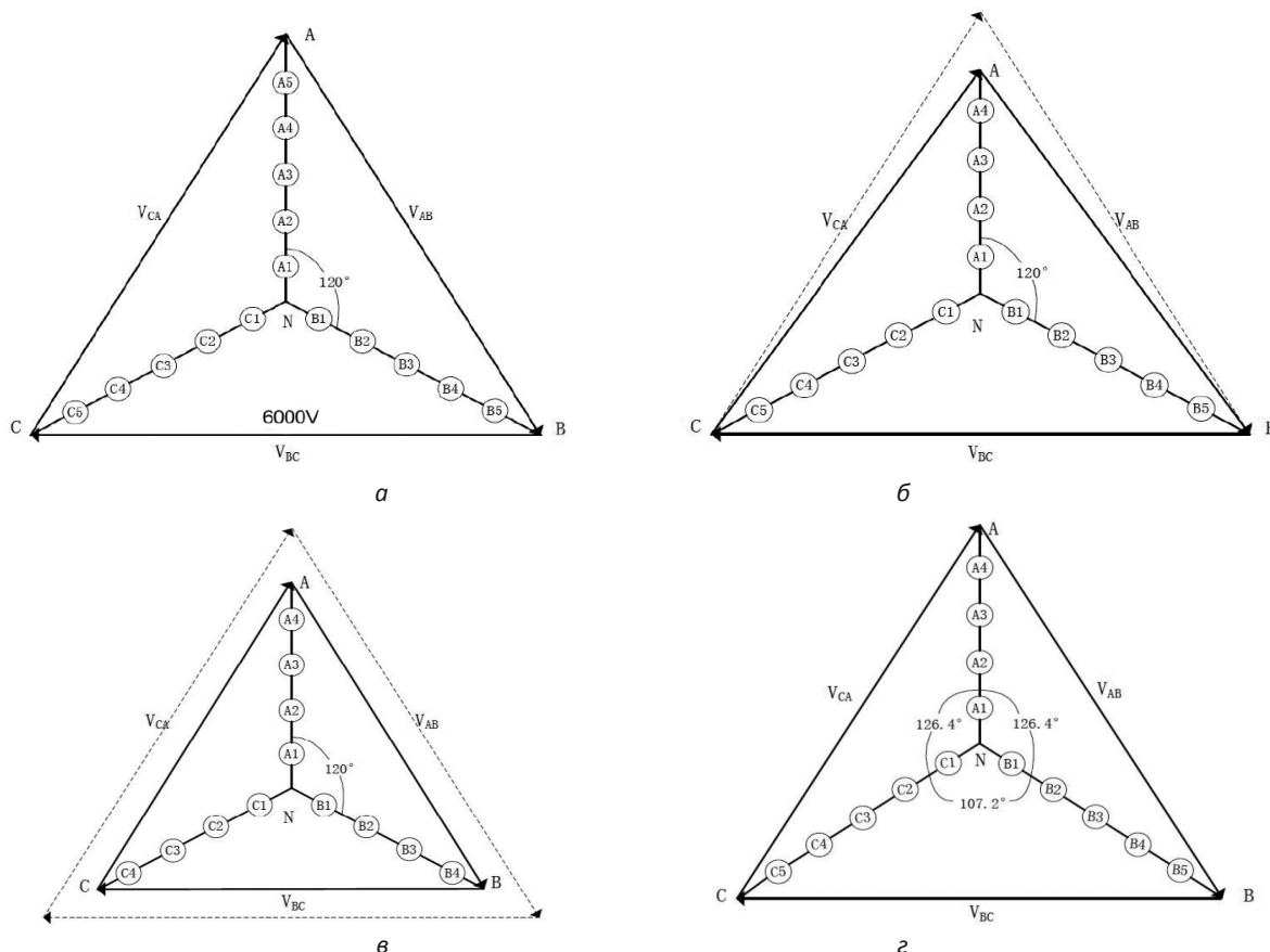
Рис. 6.2 - Диаграмма силовой части преобразователя частоты с 5 ячейками на 6 кВ
