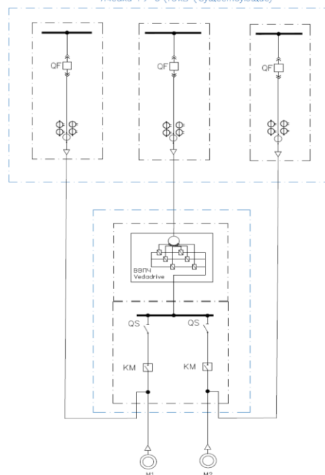
Рис. 6.6 - Схема переключения рабочий-резервный автоматический
