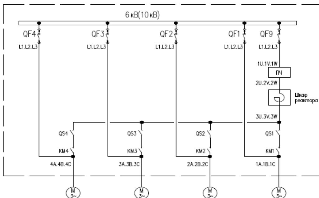
Рис. 6.13 - Схема системы «Мультистарт» на четыре двигателя с питанием от одной секции шин
