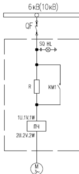
Рис. 6.11 - Силовая схема система пускового шкафа
