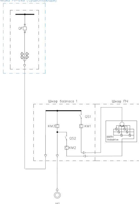
Рис. 6.4 - Схема автоматического байпаса
