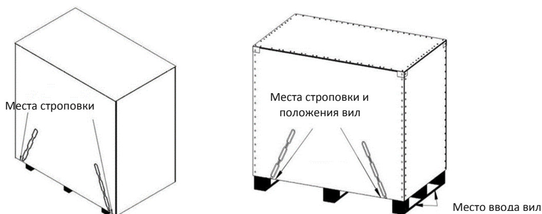
Рис. 2.5 - Строповка (паллеты с выступом - слева, паллеты без выступа - справа)
