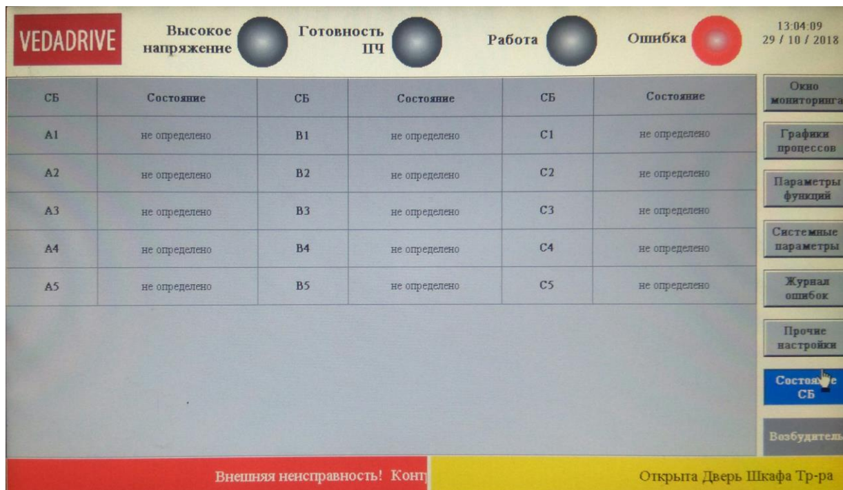
Рис. 5.12 - Окно состояния силовых ячеек
