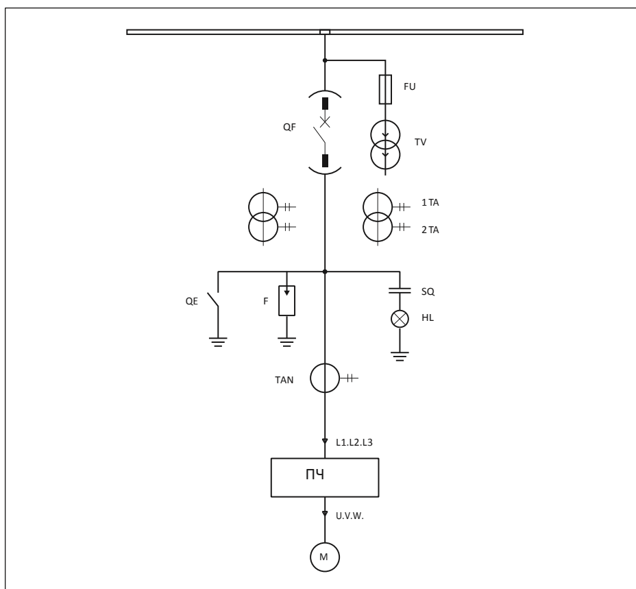
Рис. 3.1 - Электрическая схема силовой цепи
