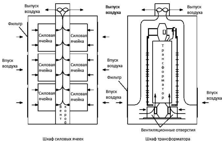
Рис. 2.2 - Стандартный вентиляционный короб преобразователя частоты 10 кВ
